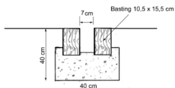
Caniveau bois pour traversées obliques
