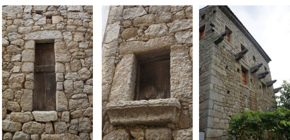
Exemple de Détails de façade
