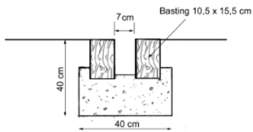
Caniveau bois pour traversées obliques
